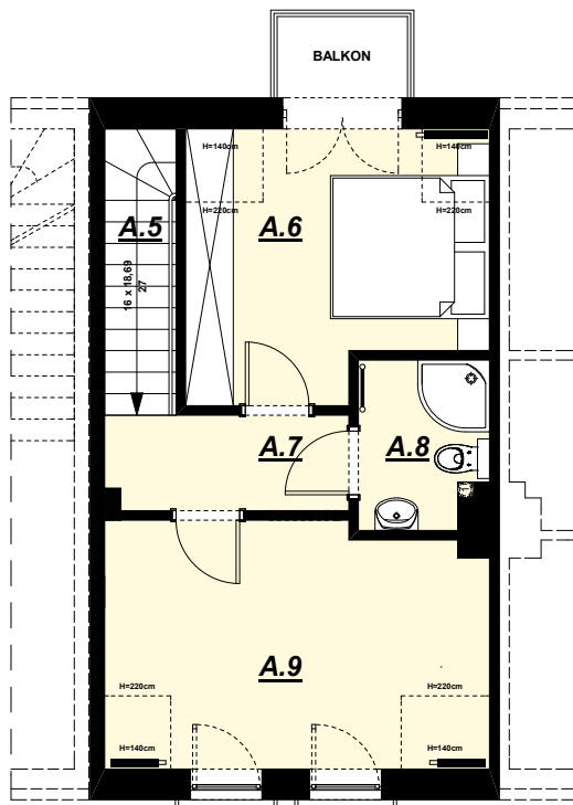
RZUT PIĘTRA
