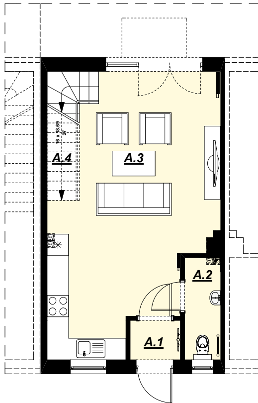
RZUT PARTERU
